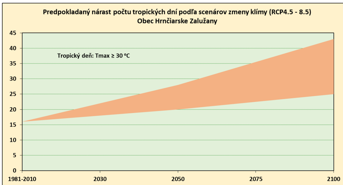
Obr.15 Predpokladaný nárast počtu tropických dní v obci Hrnčiarске Zalužany podľa RCP scenárov
